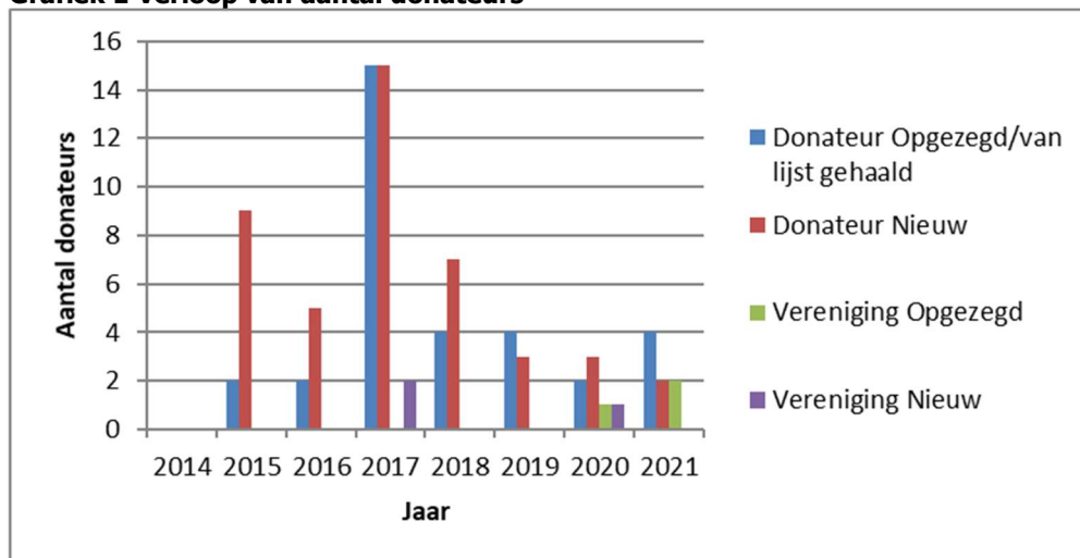
Grafiek 1 Verloop van aantal donateurs
